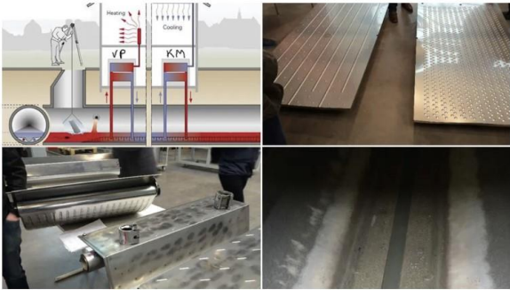
En varmepumpe/hjellemarkin er koblet mot varmevekslerelementene i avløpsrøret. Dette er det første anlegget i Norge hvor varmevekslere plasseres i selve avløpsrørnet. Bilde: Alf Bogen
